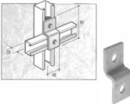
CF-22 "Z" BRACKET TOP HAT
