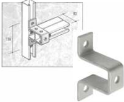
CF-27 TOP HAT
