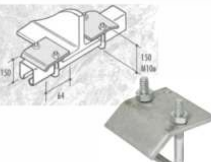
CF-46 UM BEAM CLAMP 'U'BOLT
